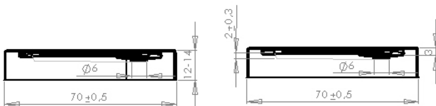
Secțiune cadita autoportanta
